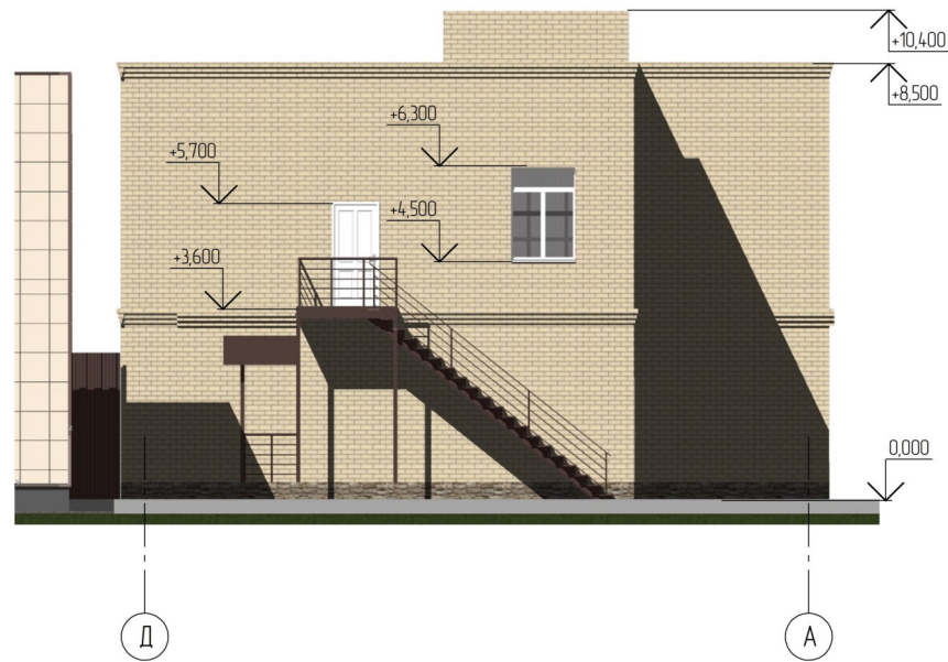
Фасад в осях Д-А
